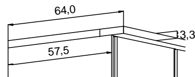
Kranzleiste
